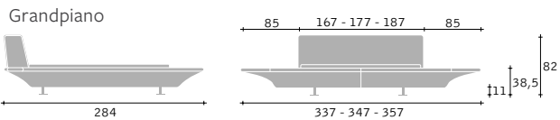
Ingombri · Outer sizes · Tamaño total · Aussenmasse · Encombrement
