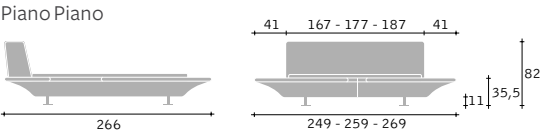
Ingombri · Outer sizes · Tamaño total · Aussenmasse · Encombrement
