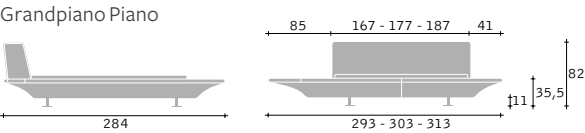
Ingombri · Outer sizes · Tamaño total · Aussenmasse · Encombrement
