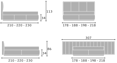
Ingombri · Outer sizes · Tamaño total · Aussenmasse · Encombrement
