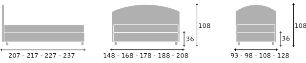
Ingombri · Outer sizes · Tamaño total · Aussenmasse · Encombrement
